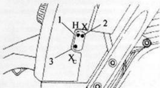
1 - регулировочный винт подачи топлива на режиме максимальной мощности; 2 - регулировочный винт подачи топлива при холостом ходе; 3 - регулировочный винт скорости холостого хода.
