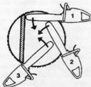
1, 2, 3 - перемещение бензопилы
