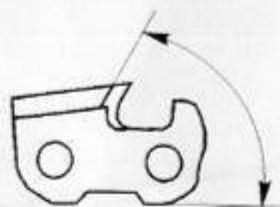
Рисунок 1.8 - Режущий угол верхней грани
