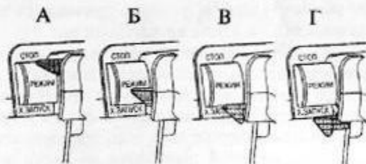
А - СТОП - положение останова, Б - РЕЖИМ - работа на холостом ходу и под нагрузкой, В - Х.ЗАПУСК вверх - Пуск в прогретом состоянии, Г - Х.ЗАПУСК вниз - Пуск в холодном состоянии Рисунок 1.14 - Режим работы двигателя
