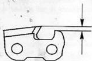
Рисунок 1.6 - Регулировка высоты ограничителя глубины пропила
