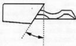
Рисунок 1.7 - Угол заточки верхней грани
