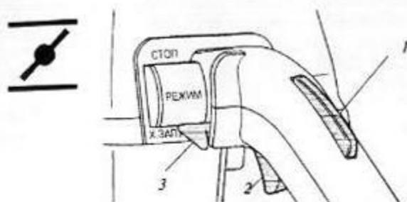
1 - стоп манетки, 2 - манетка, 3 - рычаг управления Рисунок 2.10 - Положение рычага управления и воздушной заслонки при запуске двигателя
