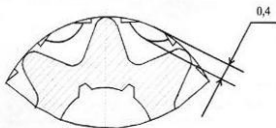
Рисунок 2.21 - Износ ведущей звездочки
