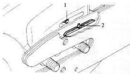
1 - маслосканал в картере, 2 - смазочное отверстие в шине Рисунок 1.11 - Смазка режущего оборудования
