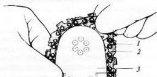
1 - цепь, 2 - ведомая звездочка, 3 - шина
