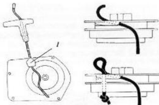
1 - люверса для шнура
