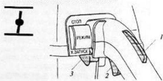
1 - стопор манетки, 2 - манетка, 3 - рычаг управления Рисунок 2.8 - Воздушная заслонка, манетка и стопор манетки в положении рычага управления Х.ЗАПУСК вниз
