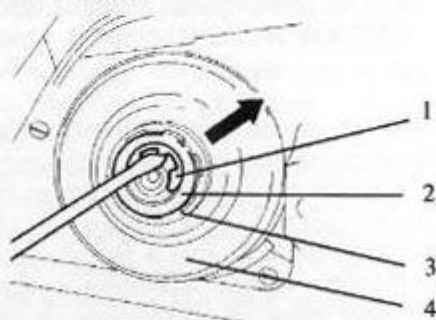
1 - упорная шайба, 2 - предохранительная шайба, 3 - ведущая звездочка, 4 - корпус полумуфты
