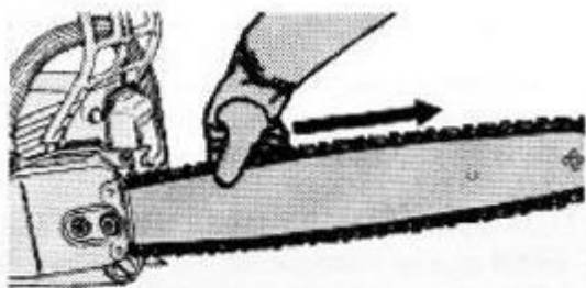
Рисунок 2.13 - Контроль натяжения пильной цепи
