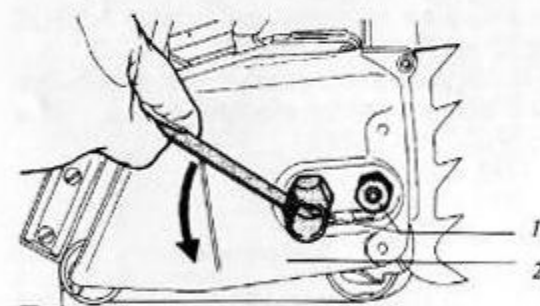
1 - шестигранные гайки, 2 - крышка правая
