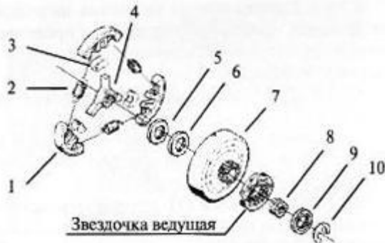
1 - сектор-груз, 2 - пружина, 3 - фиксатор, 4 - крестовина, 5 - шайба компенсационная, 6 - шайба компенсационная, 7 - корпус полумуфты, 8 - роликоподшипник, 9 - шайба предохранительная, 10 - шайба упорная
