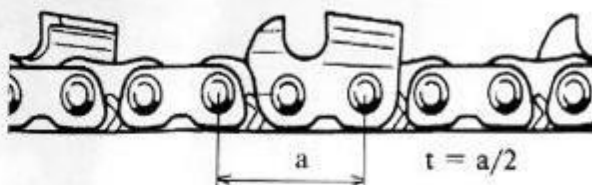
a - двойной шаг, t - шаг цепи
