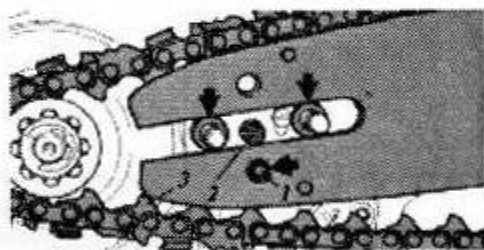
1 - штырь механизма натяжения, 2 - винт натяжения, 3 - звено пильной цепи
