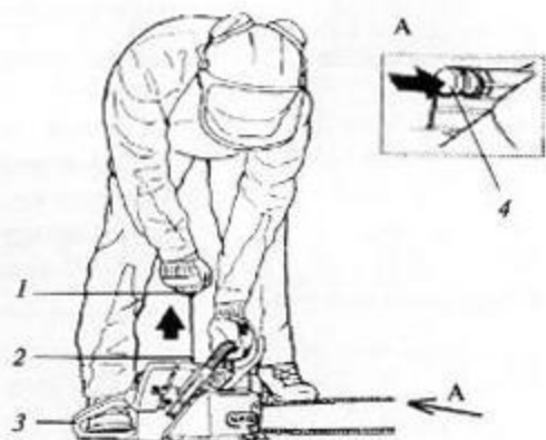
1 - рукоятка стартера, 2 - рукоятка передняя, 3 - рукоятка задняя, 4 - клапан декомпрессионный
