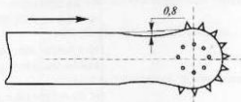
Рисунок 2.20 - Изношенный направляющий паз в районе головки шины
