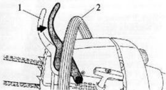
1 - рукоятка-упор (защита руки), 2 - передняя рукоятка Рисунок 1.16 - Тормоз пильной цепи отключен
