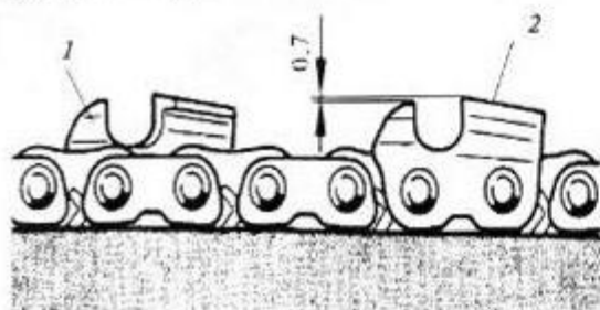
1 - ограничитель глубины, 2 - верхняя режущая грань Рисунок 2.18 - Величина глубины врезания реза
