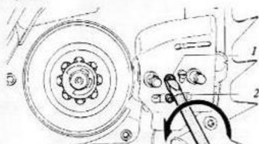
1 - винт натяжения, 2 - натяжной элемент
