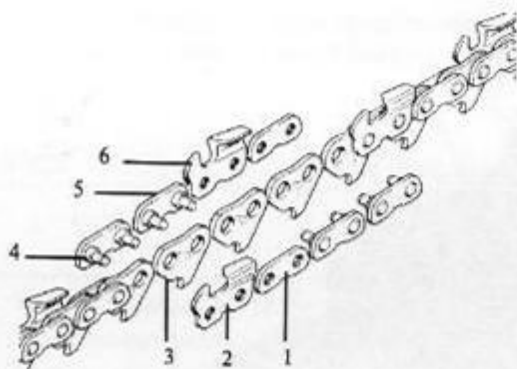
1 - соединительное звено, 2 - левое режущее звено, 3 - ведущее звено, 4 - соединительная заклепка, 5 - соединительное звено, 6 - правое режущее звено
